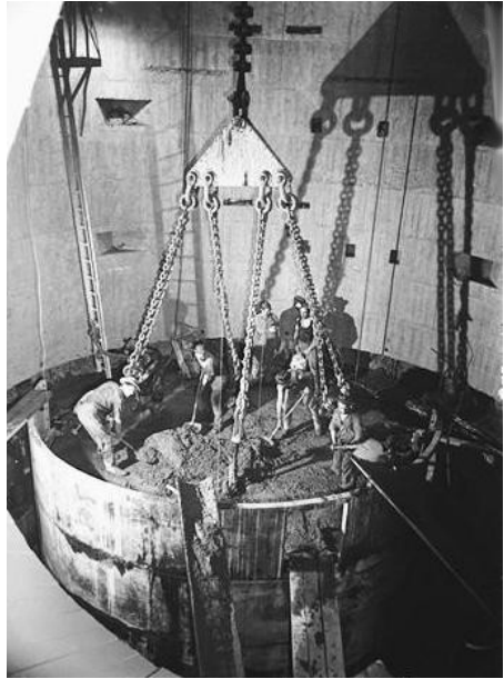
De werkvloer bij het afdiepen van de schacht
